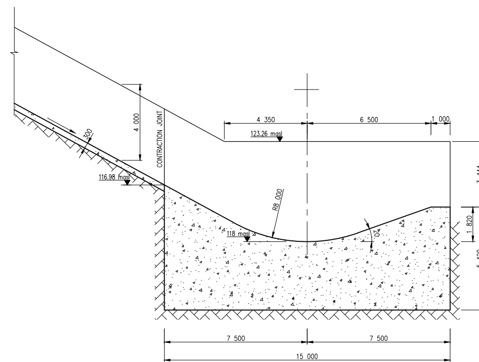
SECTION 01-01 SCALE 1 : 200
